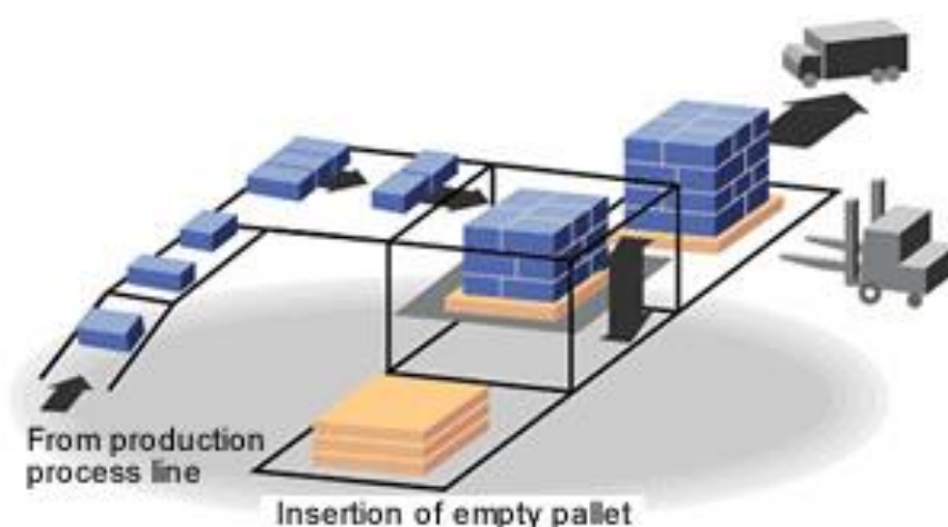
ภาพที่ 1 กระบวนการจัดเรียงกล่องสินค้าบนพาเลทด้วยเครื่อง Conventional palletizer
