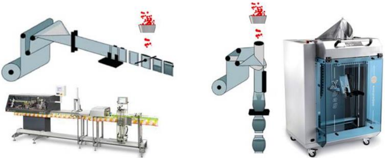
ภาพที่ 1 ตัวอย่างเครื่องบรรจุ Horizontal form-fill-seal machine และ Vertical form-fill-seal machine
