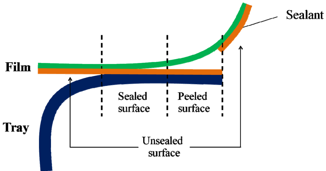
ภาพที่ 1 ลักษณะของ delamination peel
